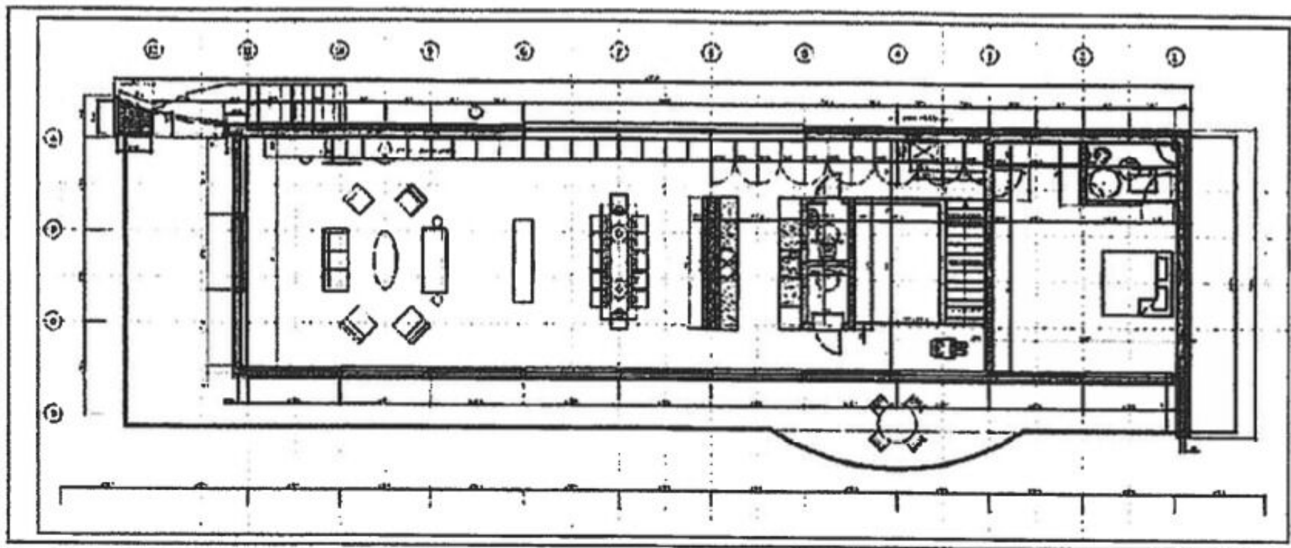
PRIMO PIANO
