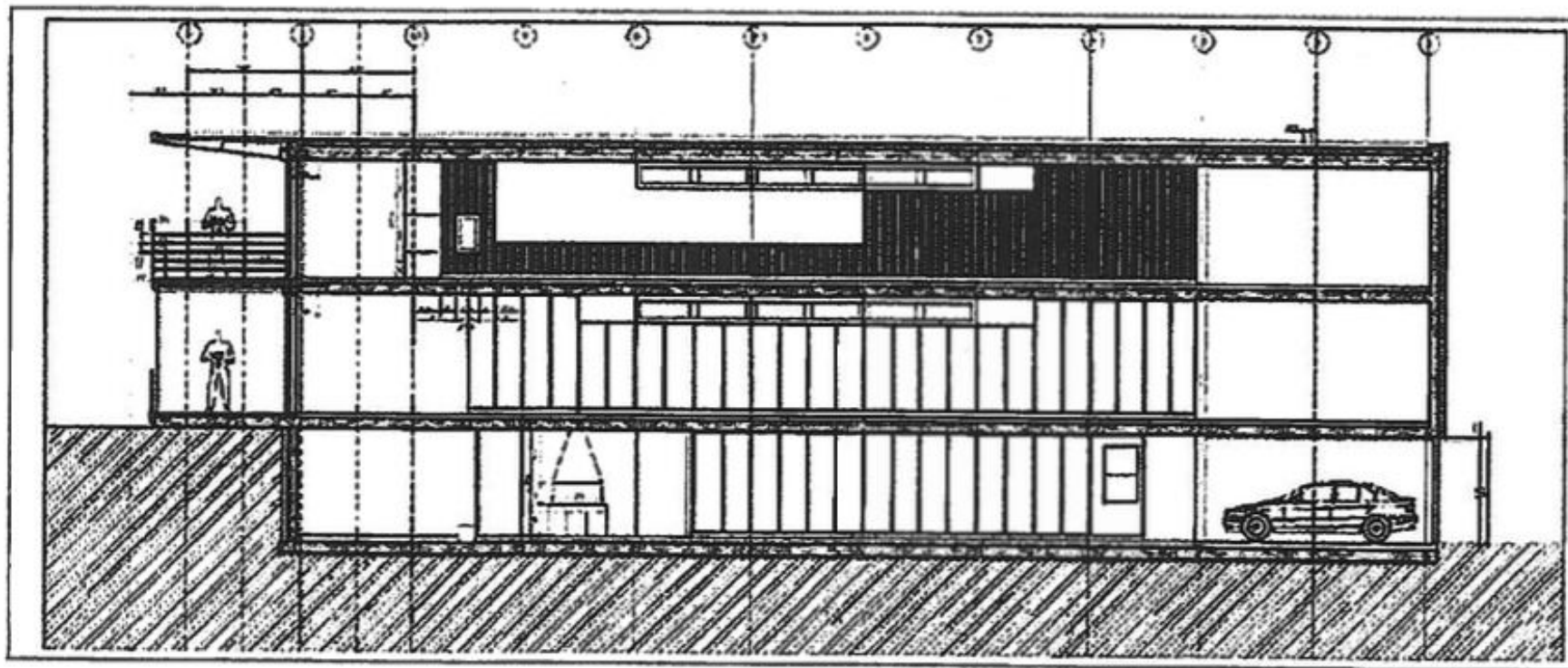
SEZIONE LONGITUDINALE
