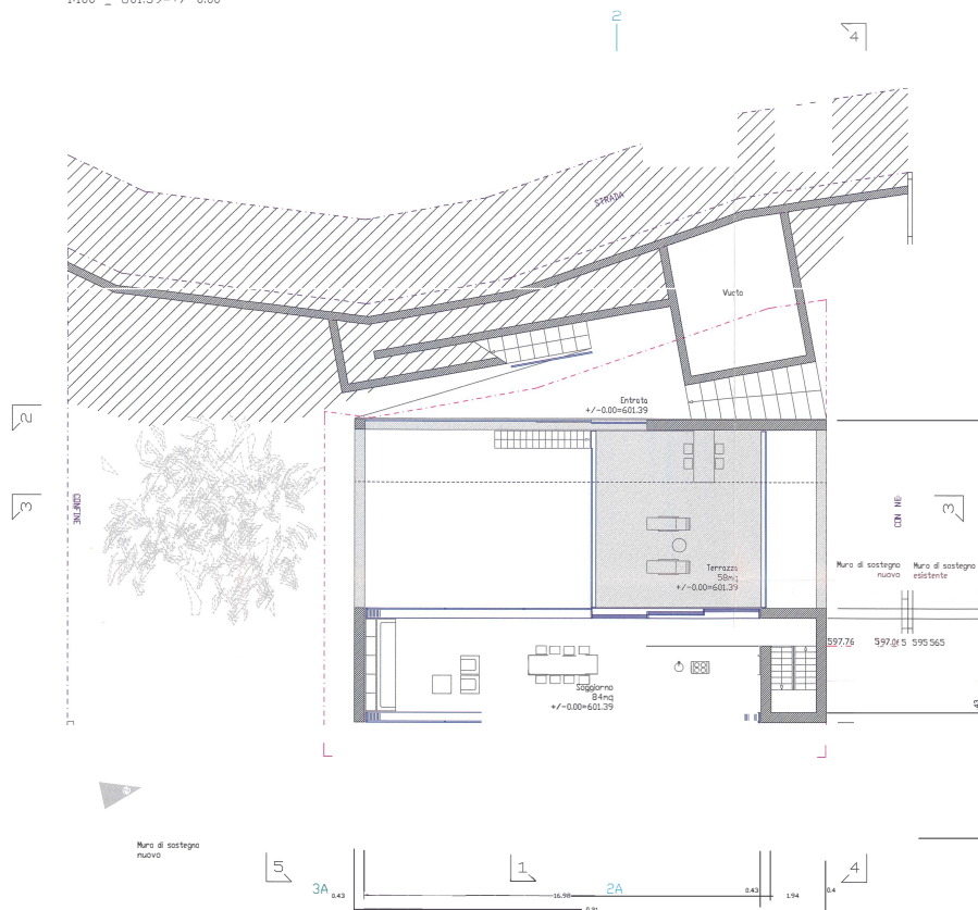
Pianta piano soggiorno 1:100 - 601.39=+/-0.00
